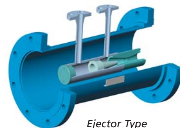
Ejector Type
