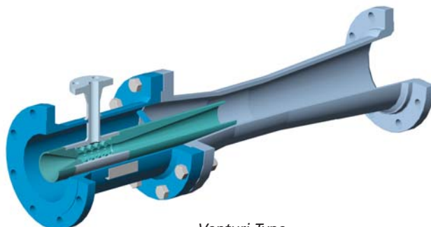
Venturi Type
